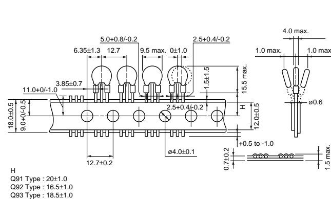
DST9_Q91/Q92/Q93
