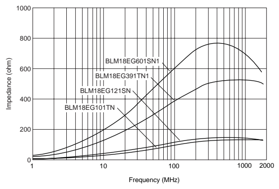
BLM18EG101TN1
