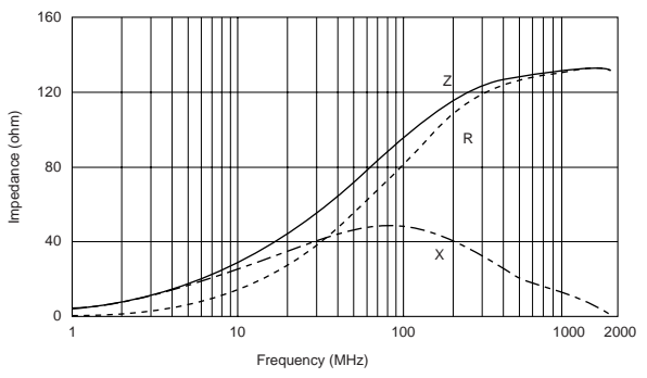
BLM18EG101TN1
