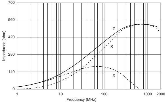
BLM18EG391TN1
